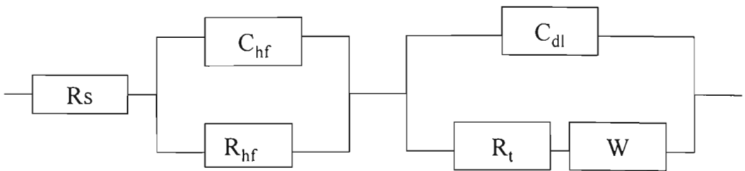
Hình 7: Sơ đồ mạch tương đương của hệ SnO_2-Sb_2O_5/Ti
