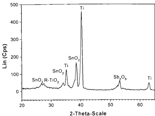
Hình 3: Giải đồ phổ nhiễu xạ tia X của màng SnO 2 tổng hợp từ dung dịch: SnCl 4 0,5 M + SbCl 3 0,5%
